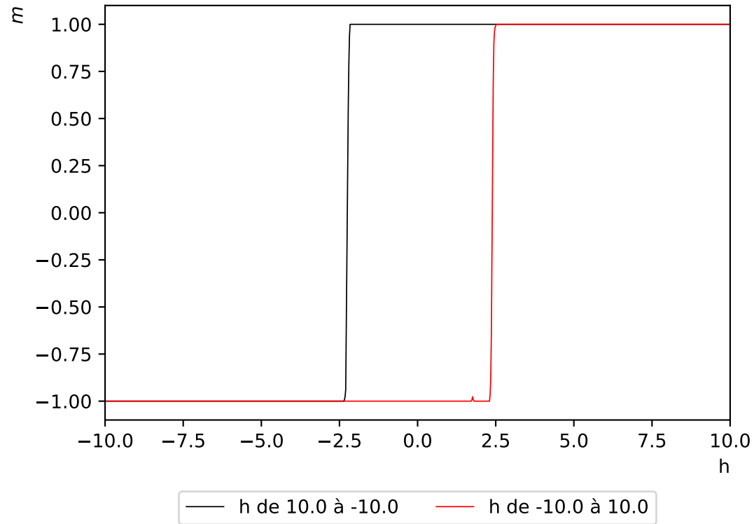
Hystérésis de l'aimantation - réseau de taille L=16 - champ magnétique d'amplitude h=10 à T=0.5
